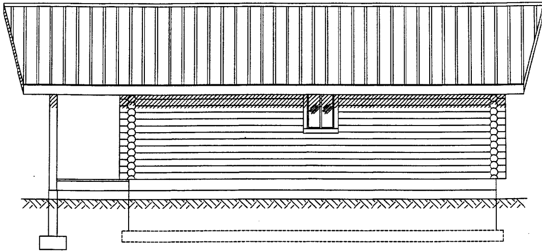
RIGHT ELEVATION
